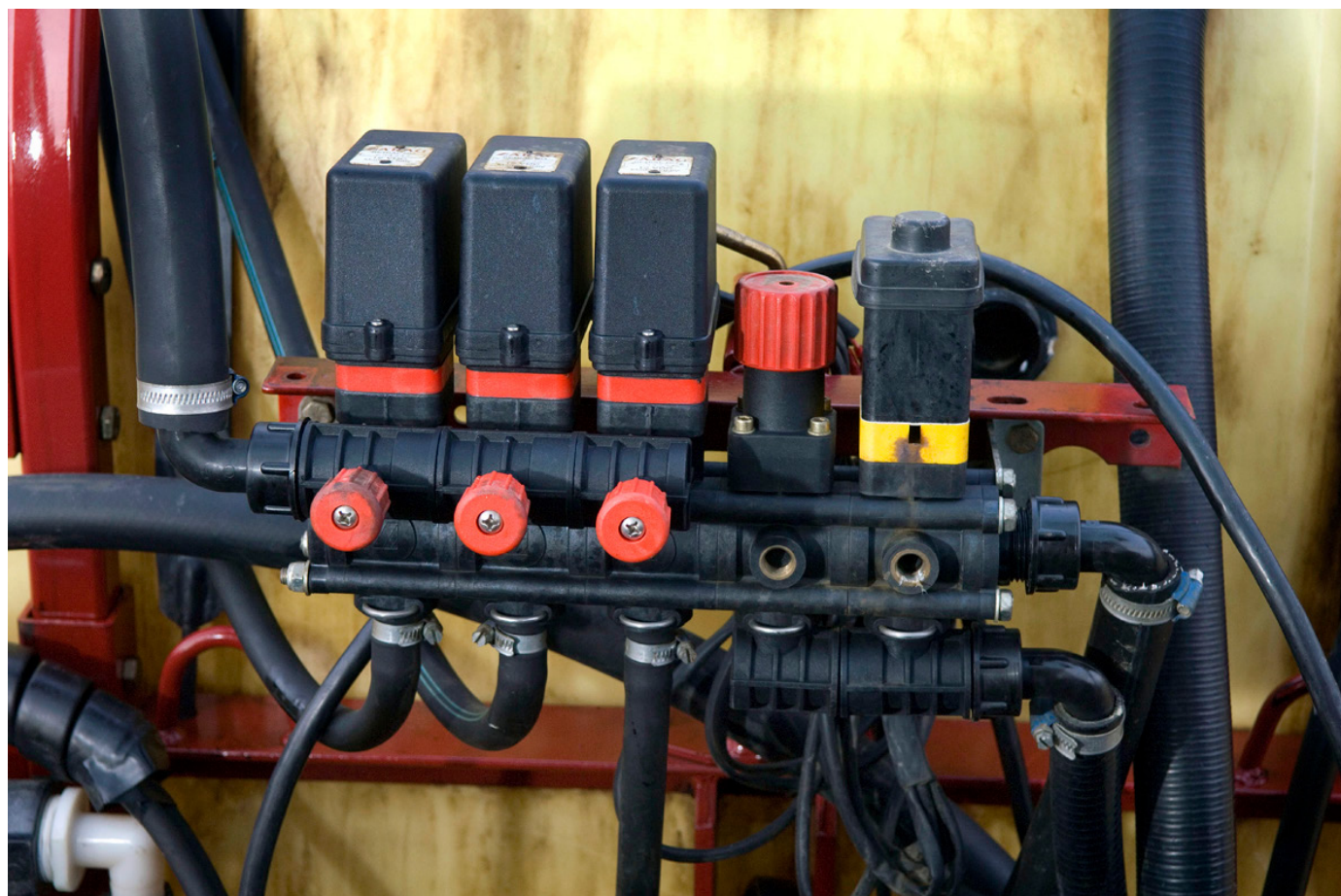
Spruta, uppgraderad med elektriska ventiler så att reglering kan ske från den stängda hytten.
