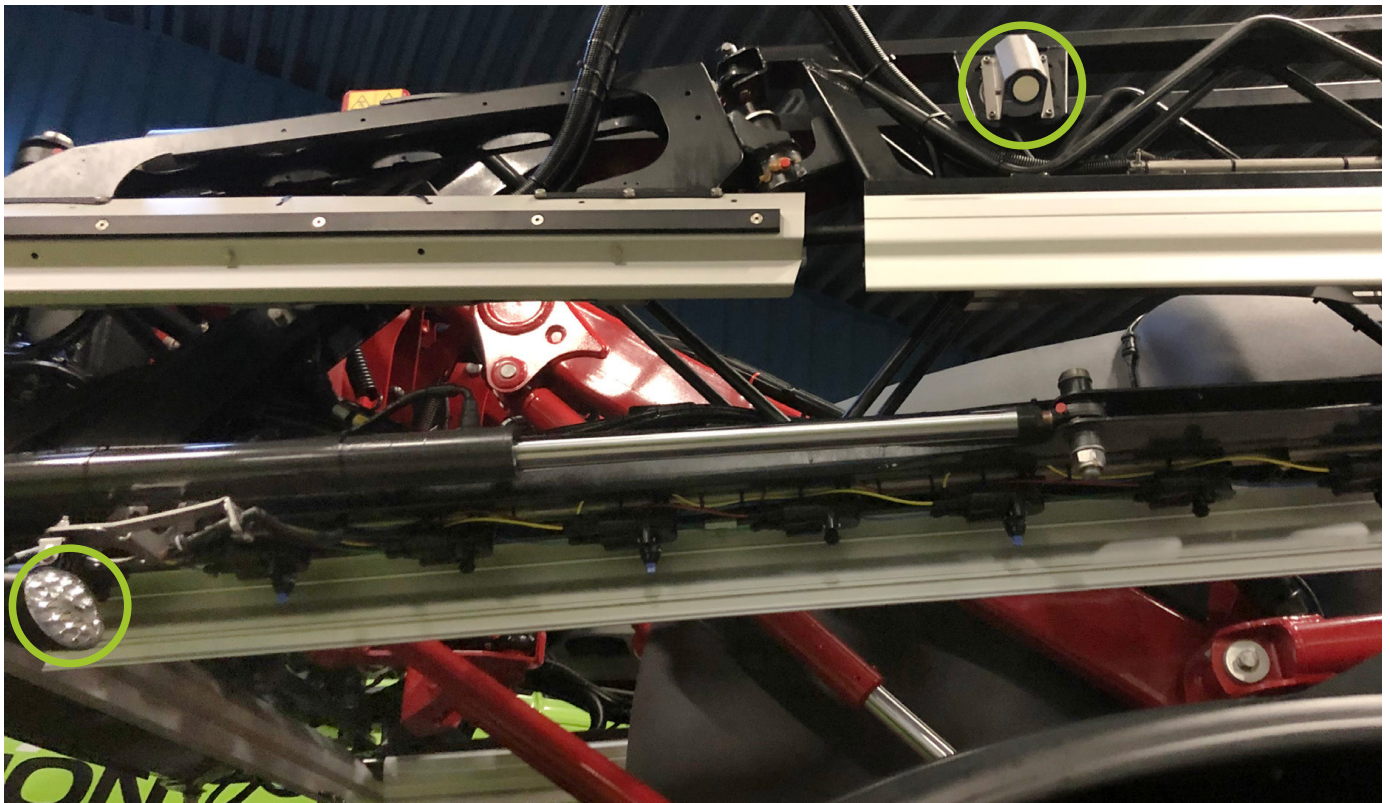
Belysning (markerad med gröna ringar i bilden) längs med rampen samt ultraljudssensor för att hålla bommen på en jämn nivå.
