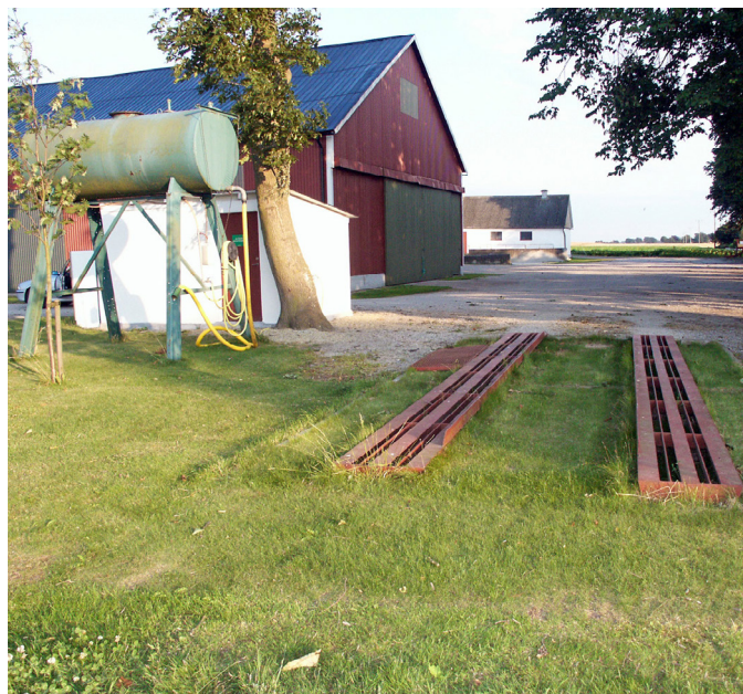
Biobädd med bra helhetslösning: Gott om plats. Vattentank för snabb påfyllning och förpackningsrengöring. Nära till förråd för mellanlagring. Biologiskt aktiv mark runt biobädden minskar riskerna ytterligare.
